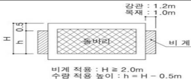
[그림 1] 비계 수량 산출 방법
